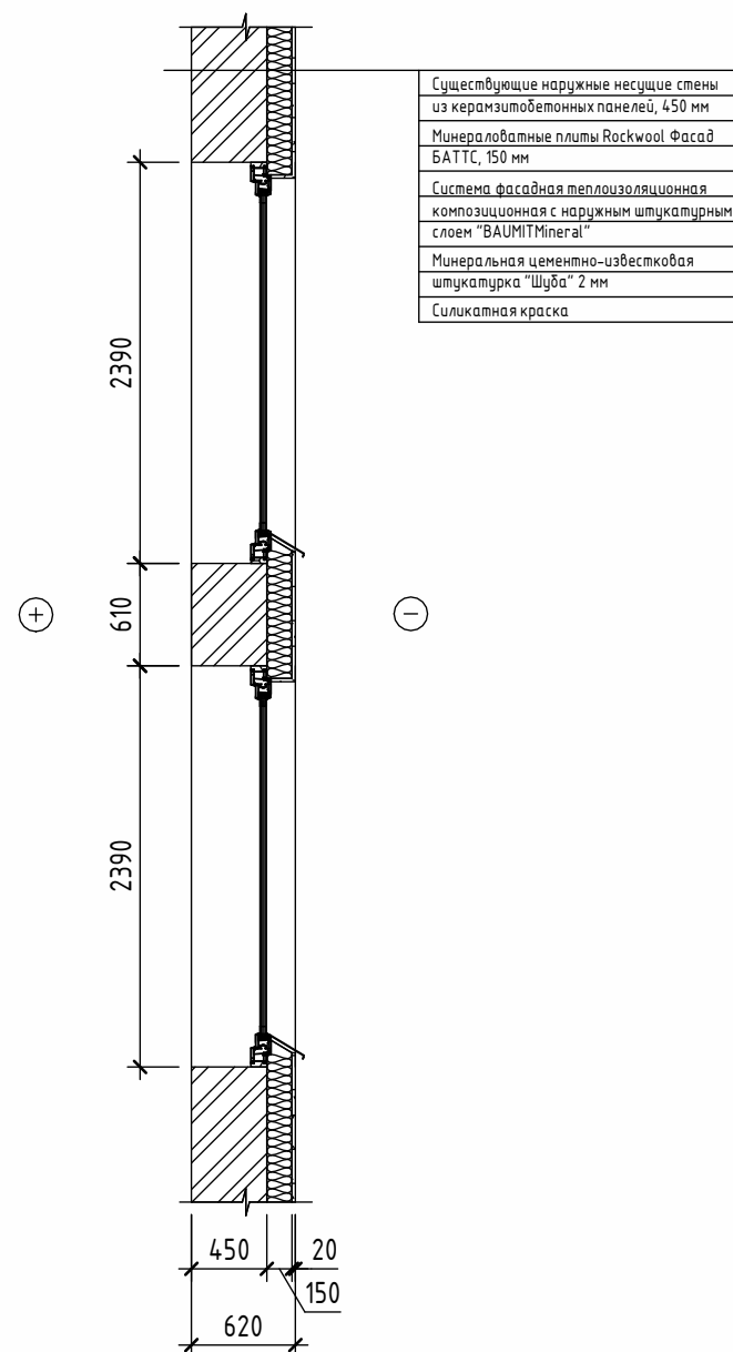
Принципиальный узел примыкания оконного блока к проему, разрез
