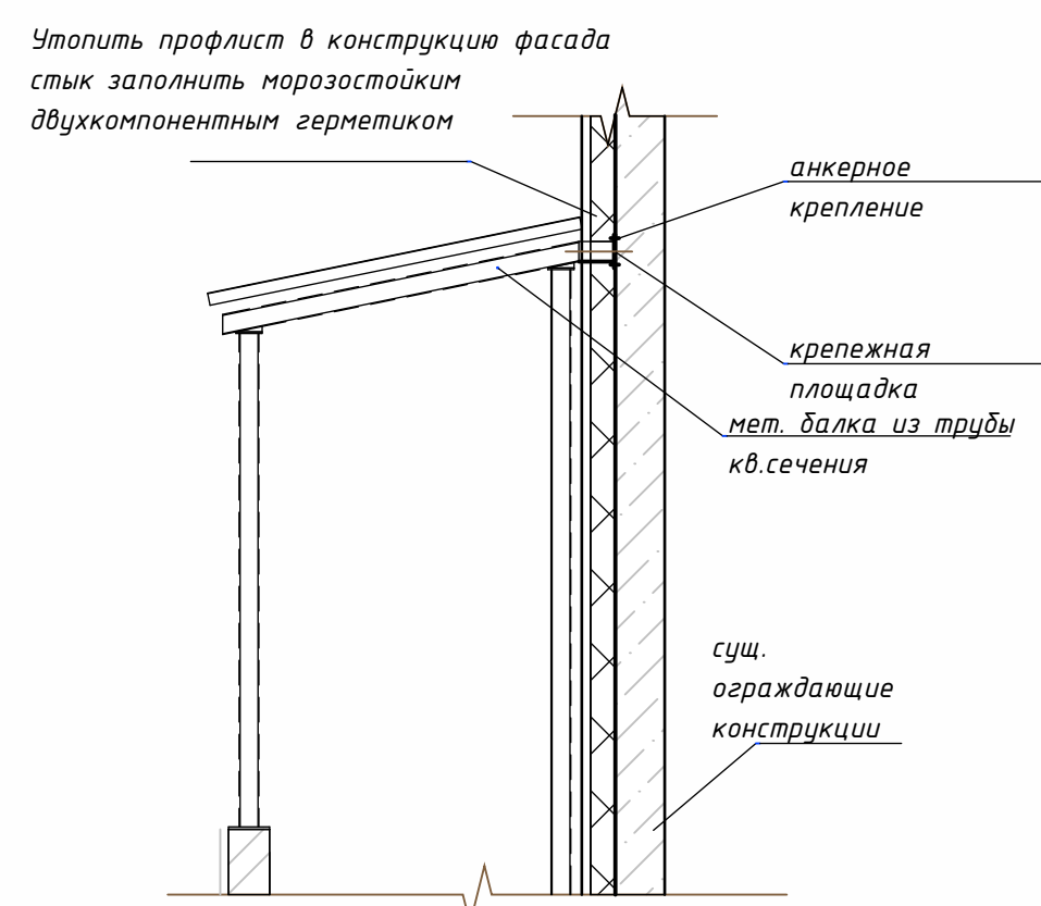
Схема крепления козырьков
