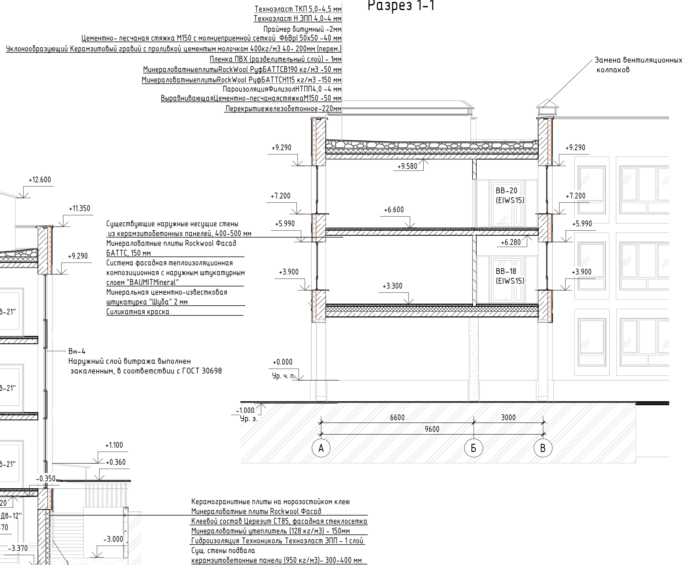
Разрез 1-1
