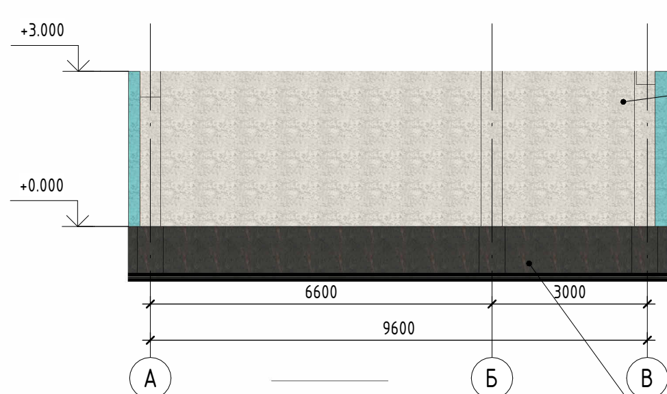
Фасад А-В по оси 6 М 1:100
