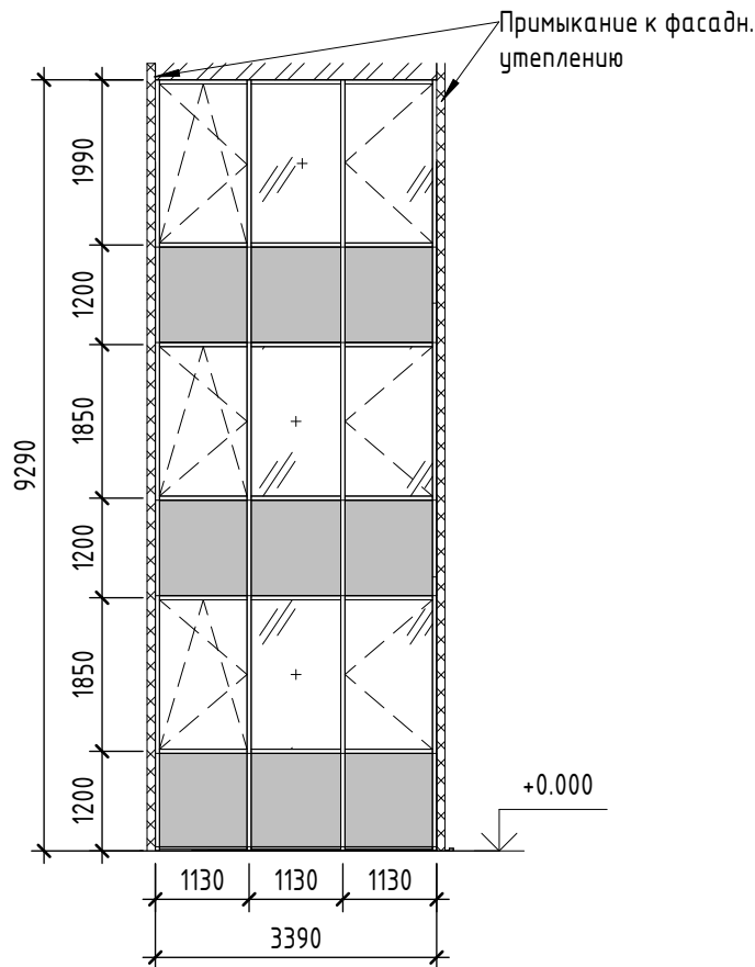
Схема витражного блока Вн-4 ( 1 : 100)
