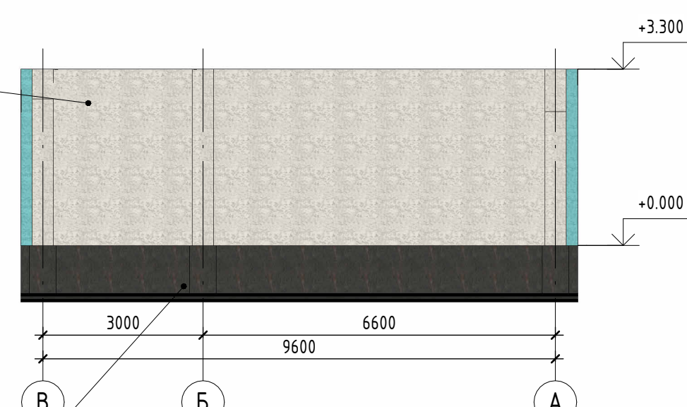
Фасад В-А по осн 17 М 1:100
