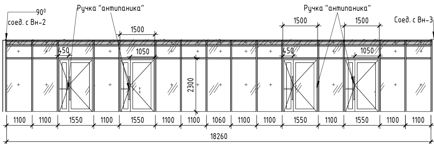
Схема витражного блока Вн-1 ( 1 : 100)
