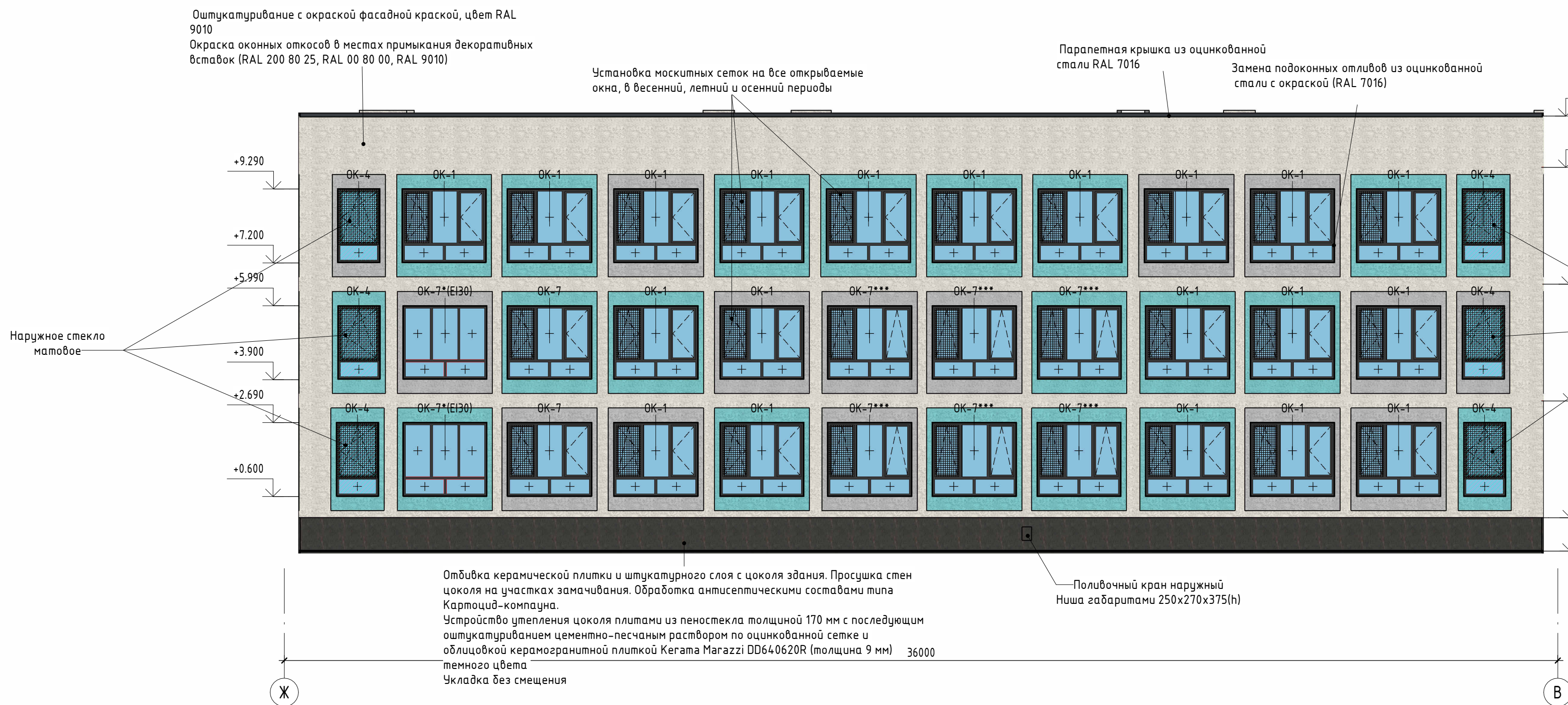
Фасад Ж-В по оси 19 ( 1 : 100)
