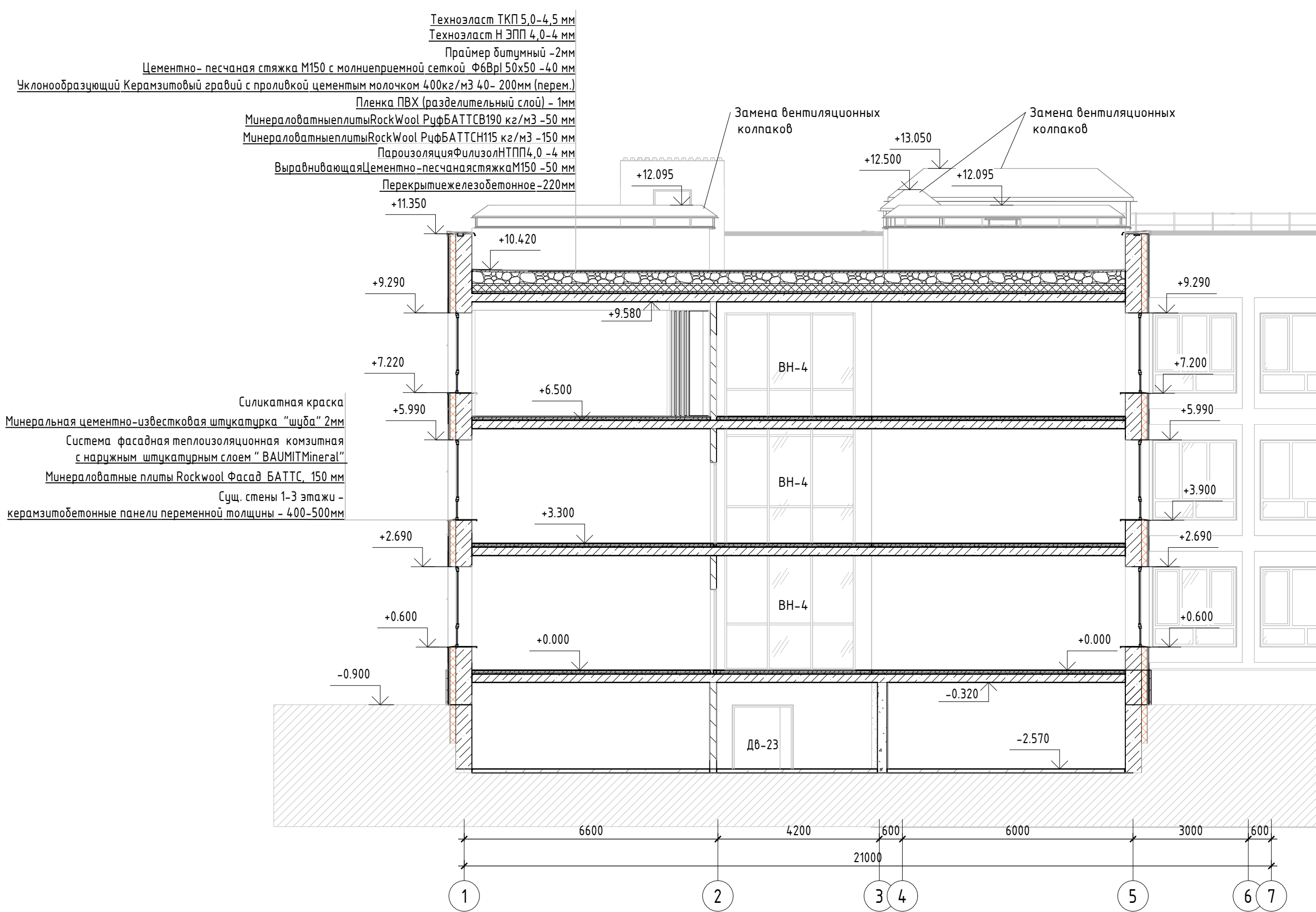
Разрез 1-1
