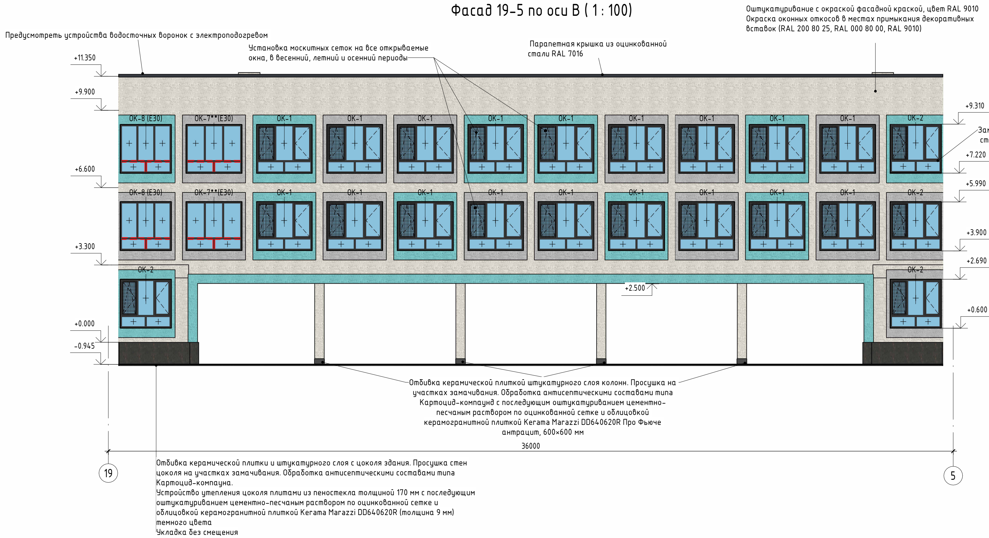
Фасад 19-5 по оси В ( 1 : 100)
