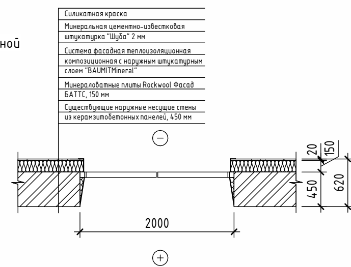
Принципиальный узел примыкания дверного блока к проему
