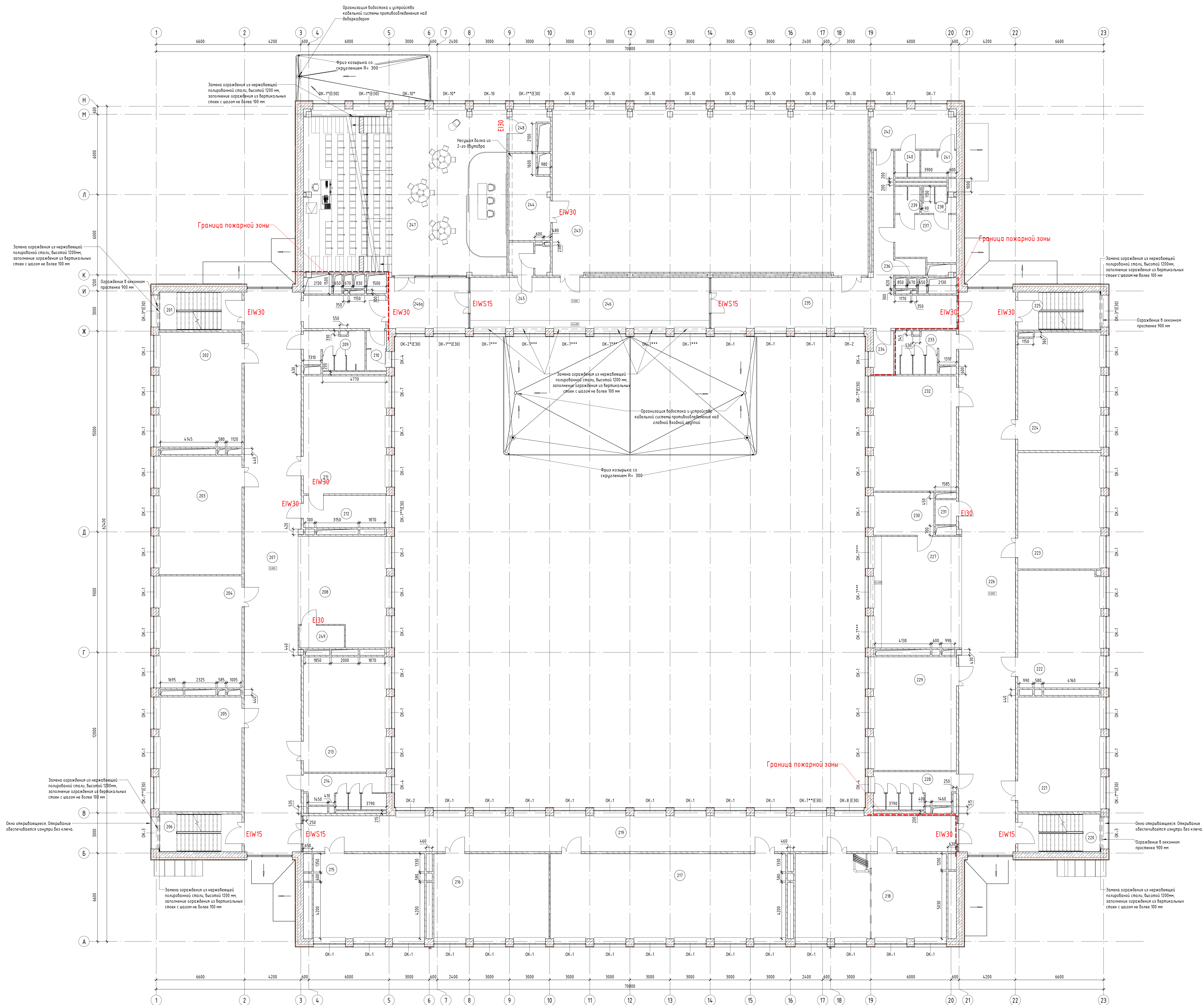
План 2-го этажа ( 1 : 100 )
