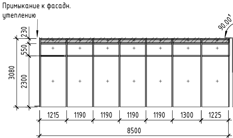
Схема витражного блока Вн-2 ( 1 : 100)
